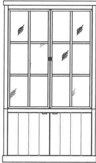
VITRINE 2 DOORS 1271 x 480 x 2200(H)
